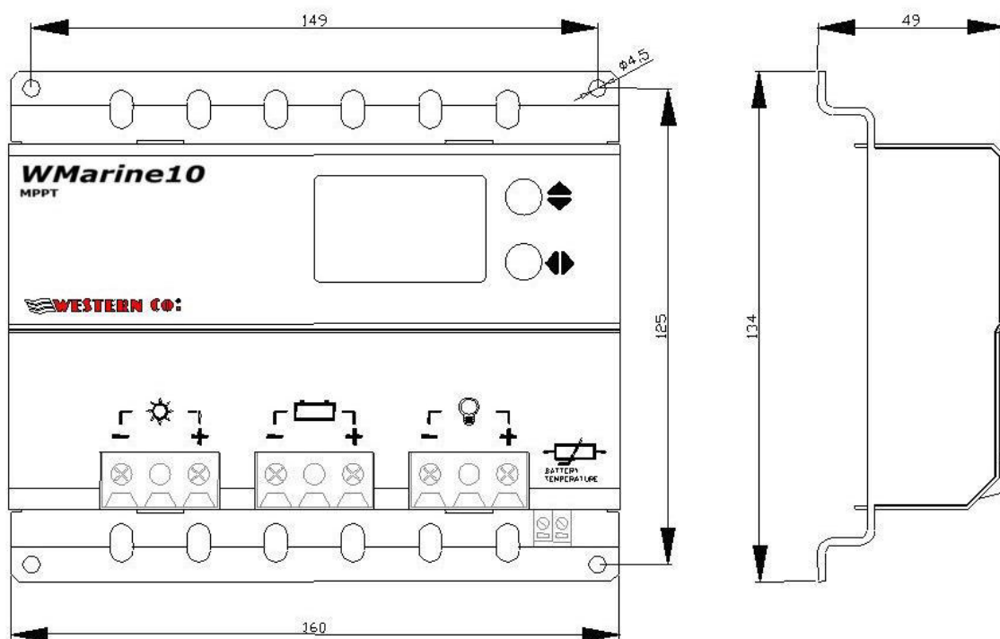
Fig.4 Dimensioni
