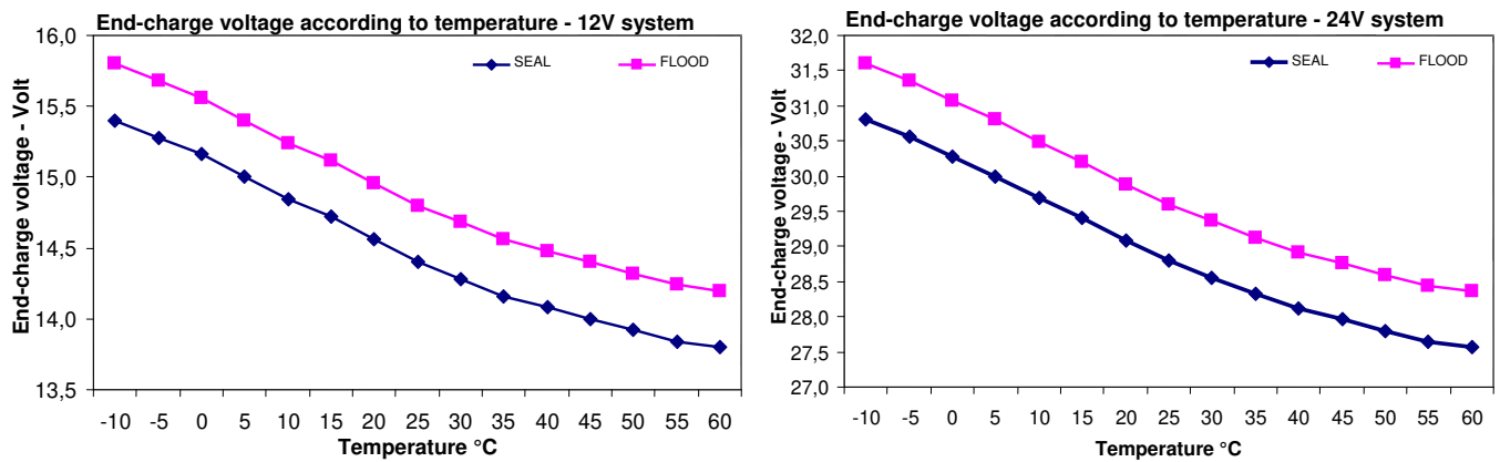
Fig.3 Curva de compensación de la tensión de recarga Veoc en función de la temperatura de batería
