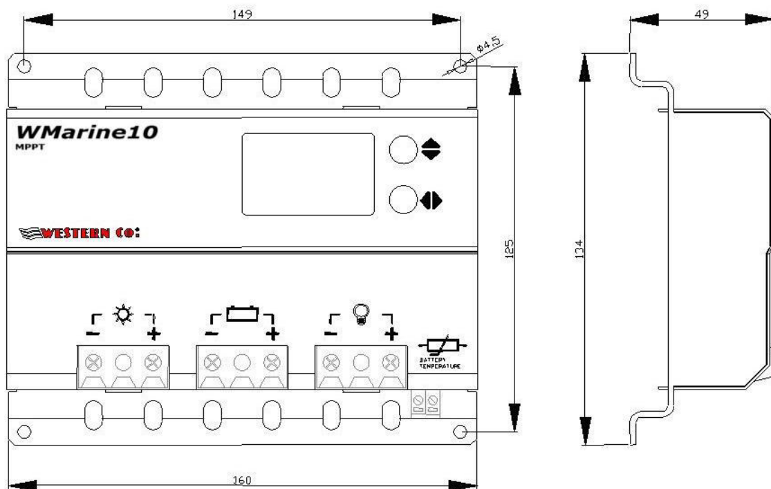
Fig.4 Dimensiones
