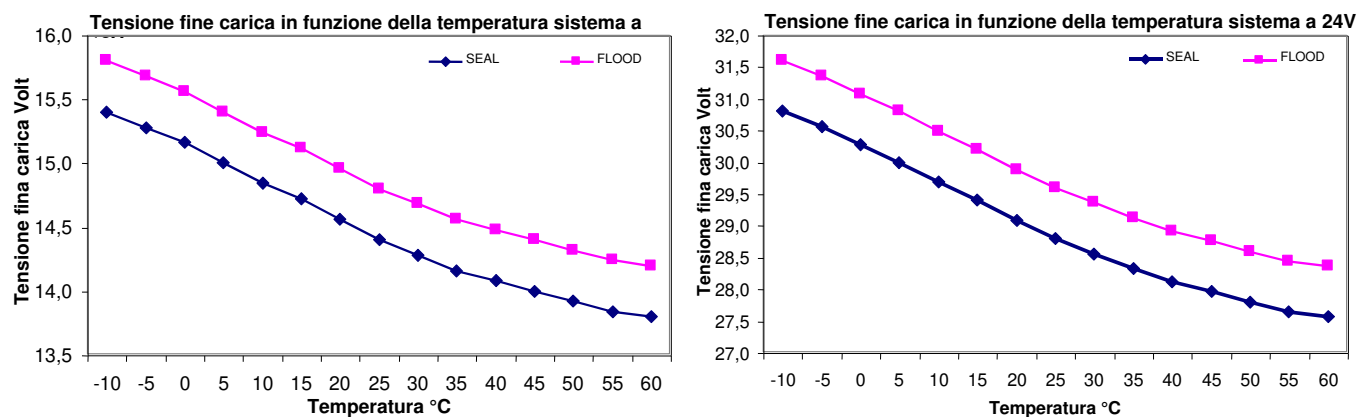
Fig.3 Curva di compensazione della tensione di ricarica Veoc in funzione della temperatura di batteria
