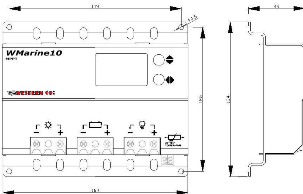
Pic.4 Dimensions
