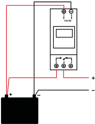
Normalmente abierto (NO)
