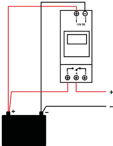
Normalement ouvert (NO)
