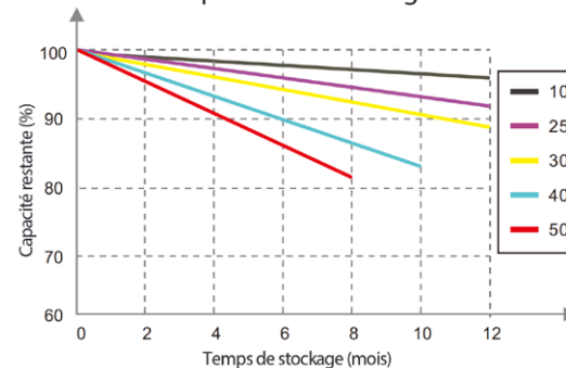
Caractéristiques d'auto-décharge
