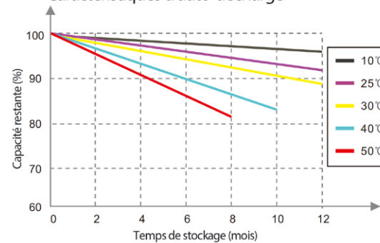
Caractéristiques d'auto-décharge
